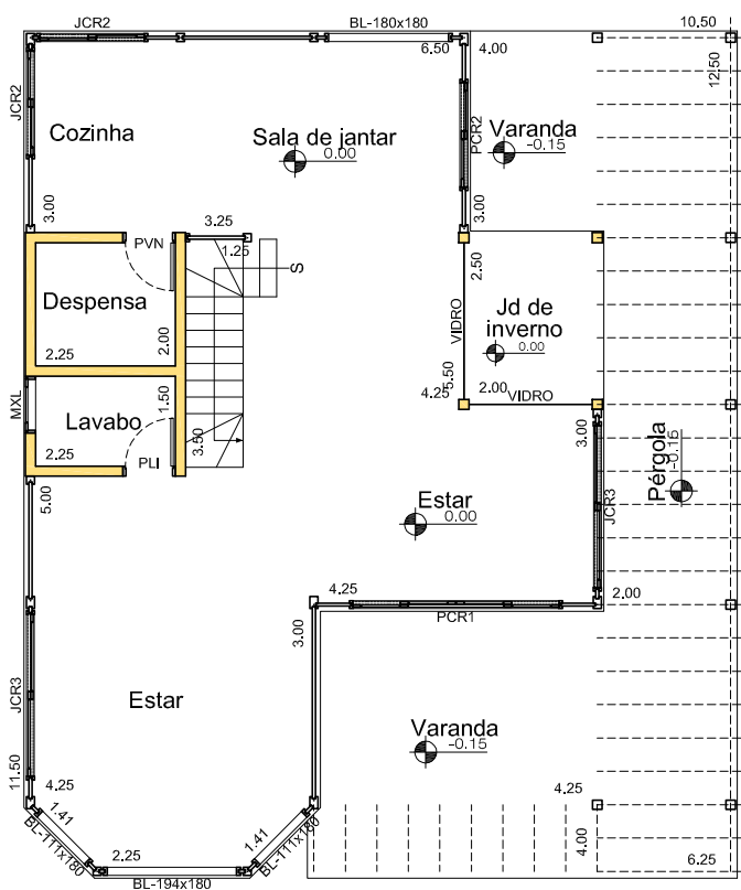
Planta baixa - Térreo
