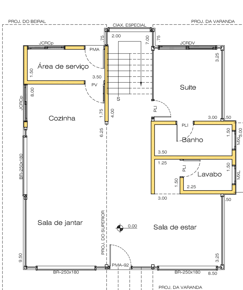
Planta baixa - Térreo
