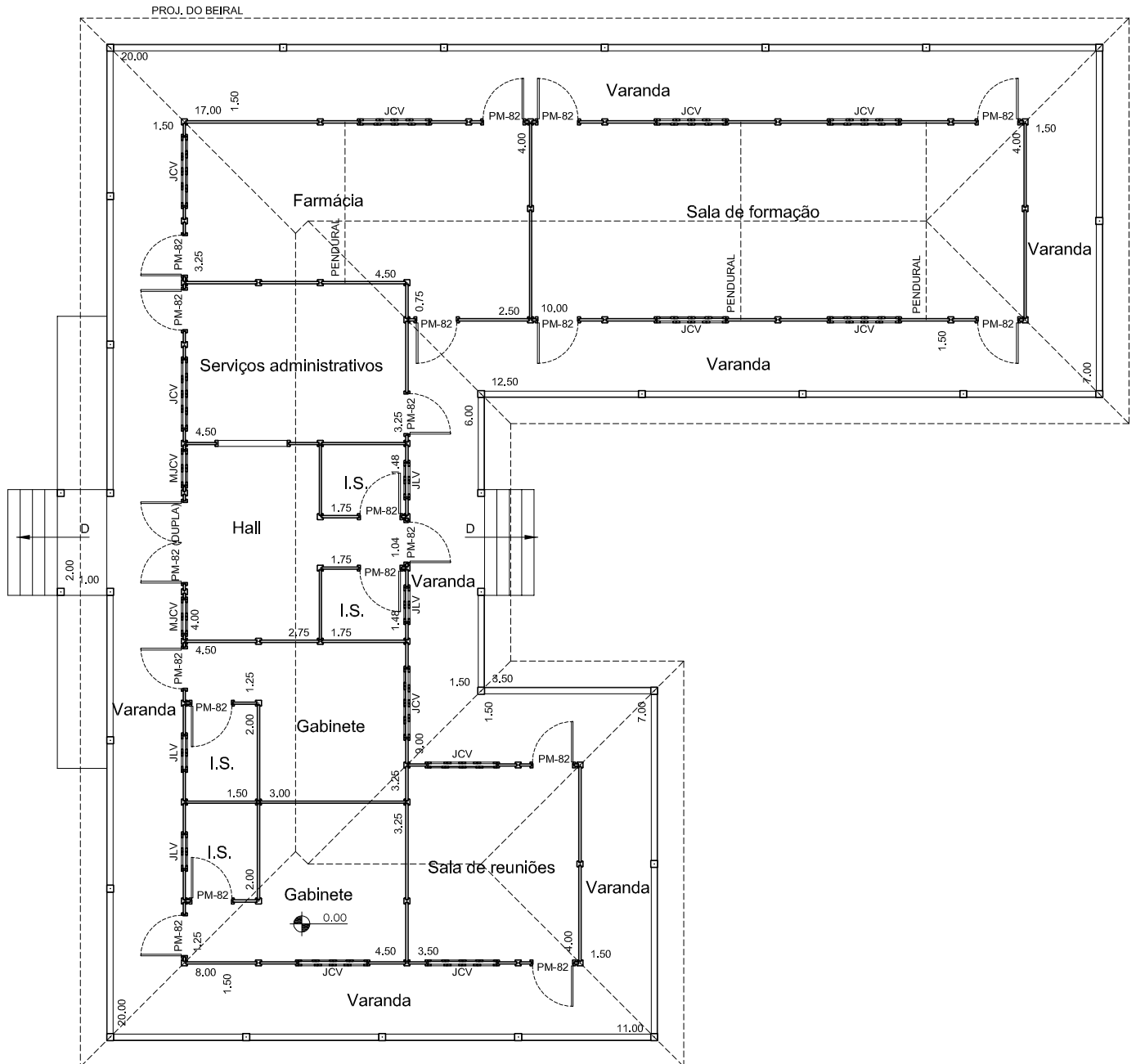
Planta baixa - Bloco de serviços administrativos
