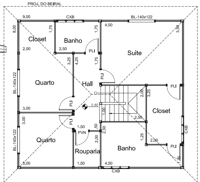
Planta baixa - Superior
