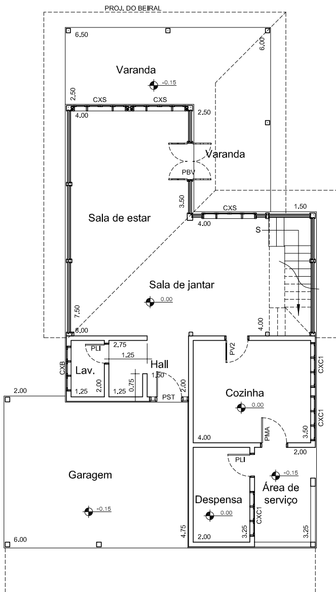
Planta baixa - Térreo Escala = 1:125
