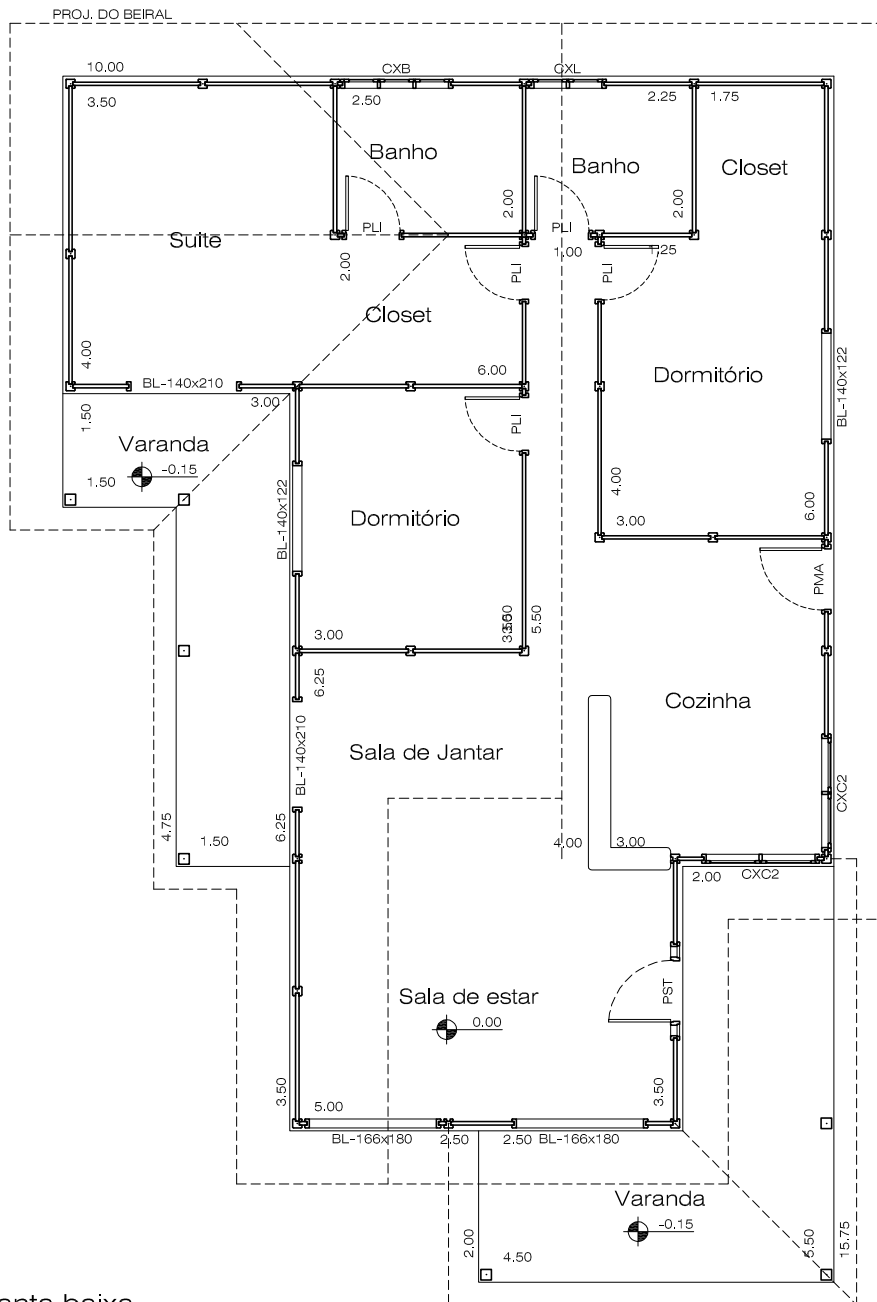
Planta baixa
