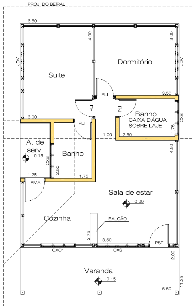
Planta baixa
